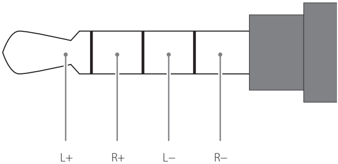
Kopplingsschema
